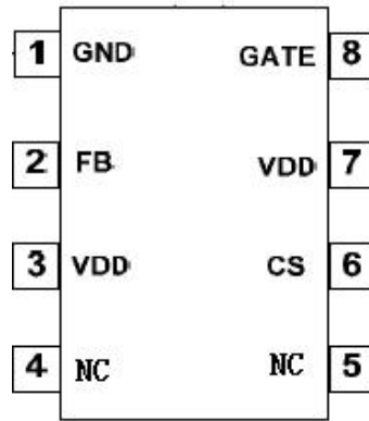
SOP8
