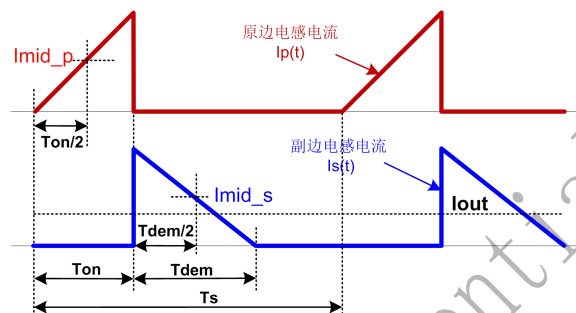
断续模式下反激电源波形
