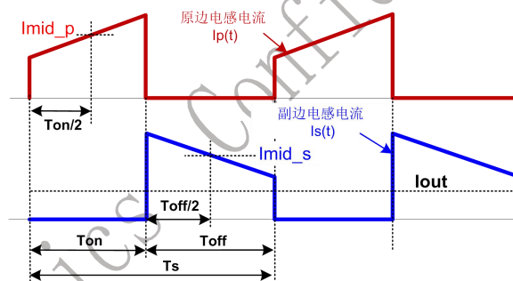
连续模式下反激电源波形
