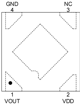
DFN4L 封装
