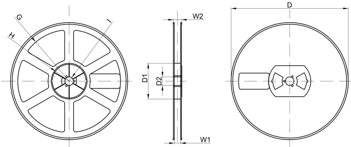
SOT23-3 卷盘
