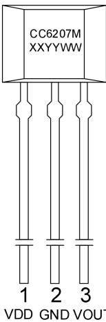
TO-92S 封装
