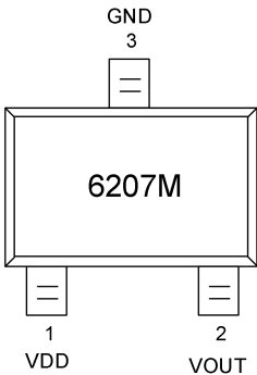
SOT23-3 封装
